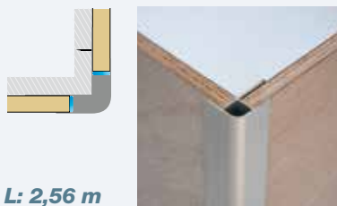
② Buitenhoek / Profilé d'angle extérieur
