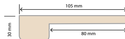
Lambriseringslijst / L: 2,56 m Moulure Lambris
