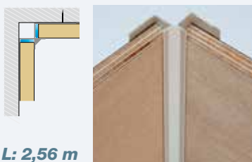
① Binnenhoek / Profilé d'angle intérieur
