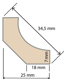
Hollijst / L: 2,5 m Moulure creuse
