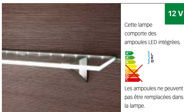
Etagère en verre éclairée 520* | Titane 249 | 1,5 watt Support d'étagère* | Aluminium anodisé | 130 x 61 x 20 mm
