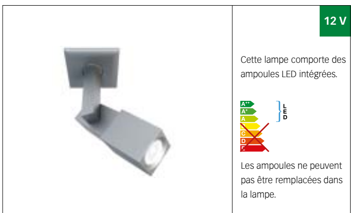
Lampe incorporée LED BT Apollo-Quadro | 5 watts | pivotable 350° et orientable 90° | focalisation possible du projecteur à lumière diffuse
