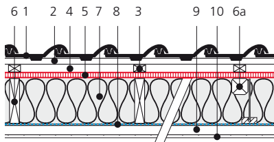
isolation entre les chevrons (nouvelle construction / rénovation)
