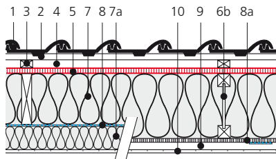
isolation avec limitation accrue des ponts thermiques
