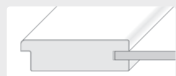
Rahmentürkonstruktion mit eingesetzten Füllungen, Rahmenfrieze aus MDF
